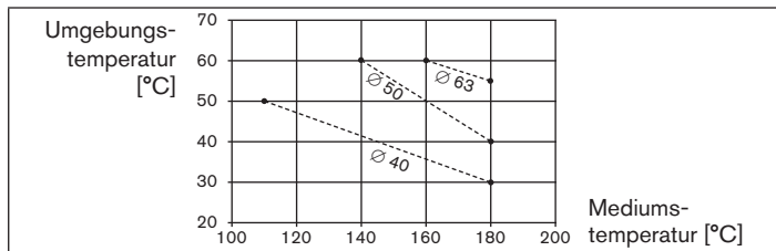
Bild 5: Temperaturbereich der maximalen Mediustemperatur und Umgebungstemperatur bei PA Antrieben
