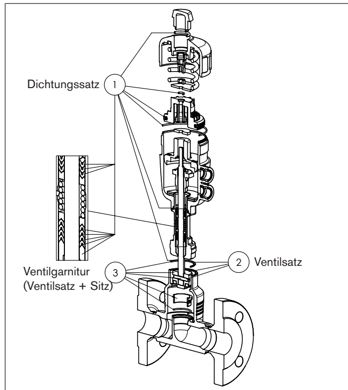
Bild 22: Übersicht Ersatzteile
